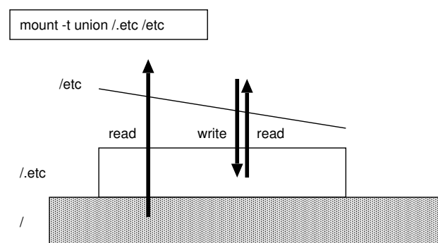
図 1 unionfs の概要
